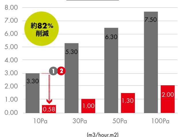
VKP®ベーシックを施工した樹脂サッシ
