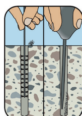
2.下穴内部の削り屑を除去
