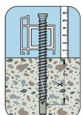
3.位置を調整しサッシを取り付ける
