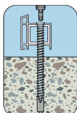
4.ネジを閉める
